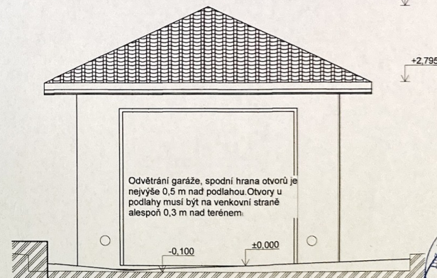
P3 Pohled Severní (4) 1:50
