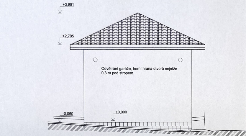
P1 Pohled Jižní 1:50
